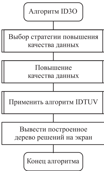
Рис. 1. Алгоритм ID3O
