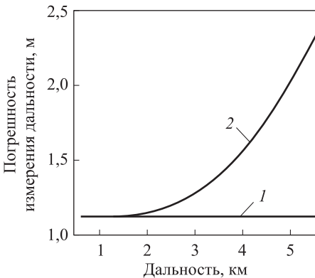
Рис. 2. Зависимость от дальности суммарной погрешности измерений ЛЛС:
