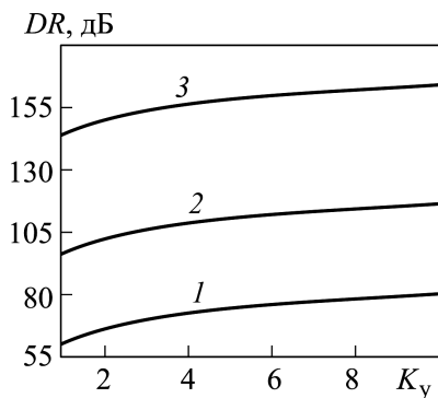
Рис. 7. Зависимость динамического диапазона преобразователя от коэффициента предварительного усиления для 10- (1), 16- (2), и 24-разрядного (3) преобразователя
