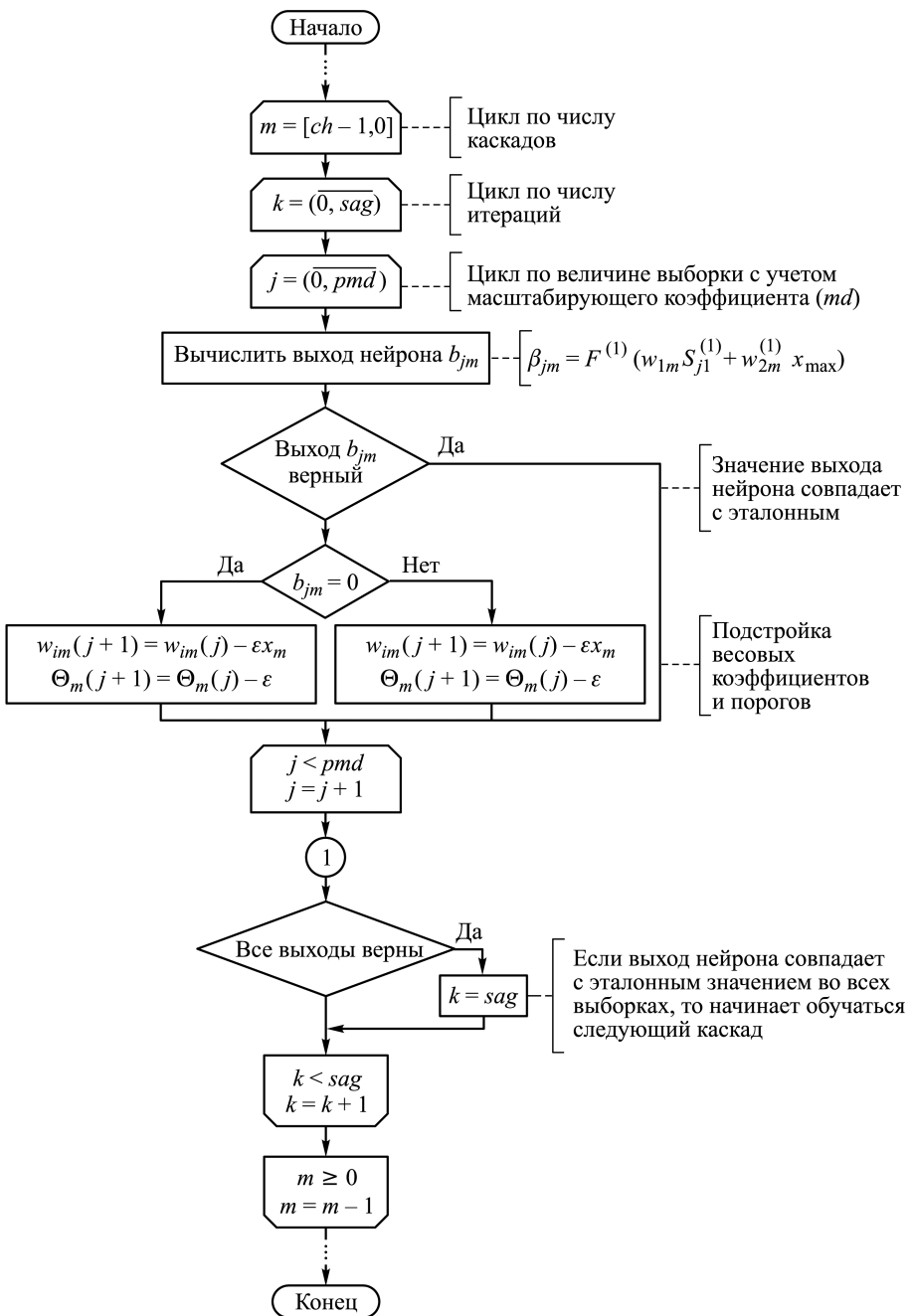
Рис. 3. Алгоритм обучения сети преобразователя U \rightarrow N_j :
