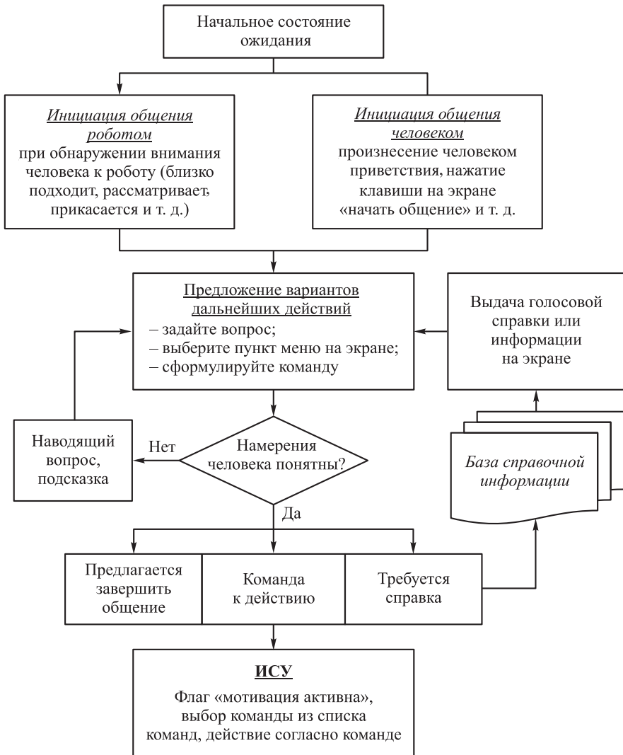
Рис. 3. Схема алгоритма функционирования интерфейса АМСП–человек
